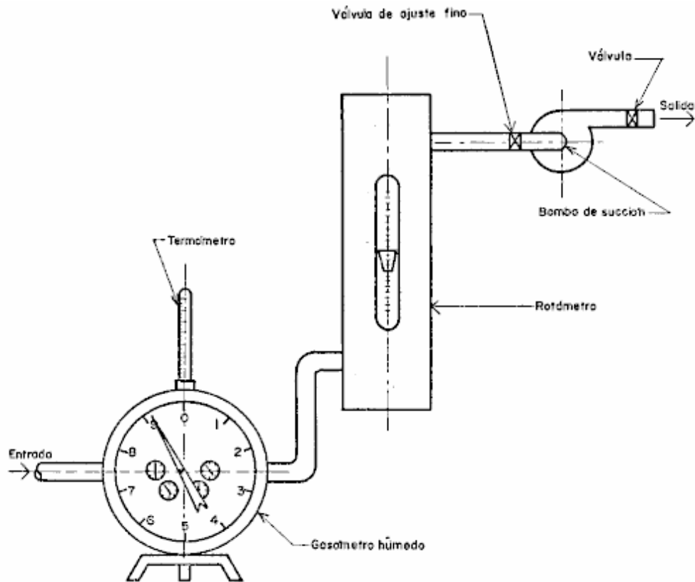
FIGURA 1.- SISTEMA DE CALIBRACION DEL ROTAMETRO
