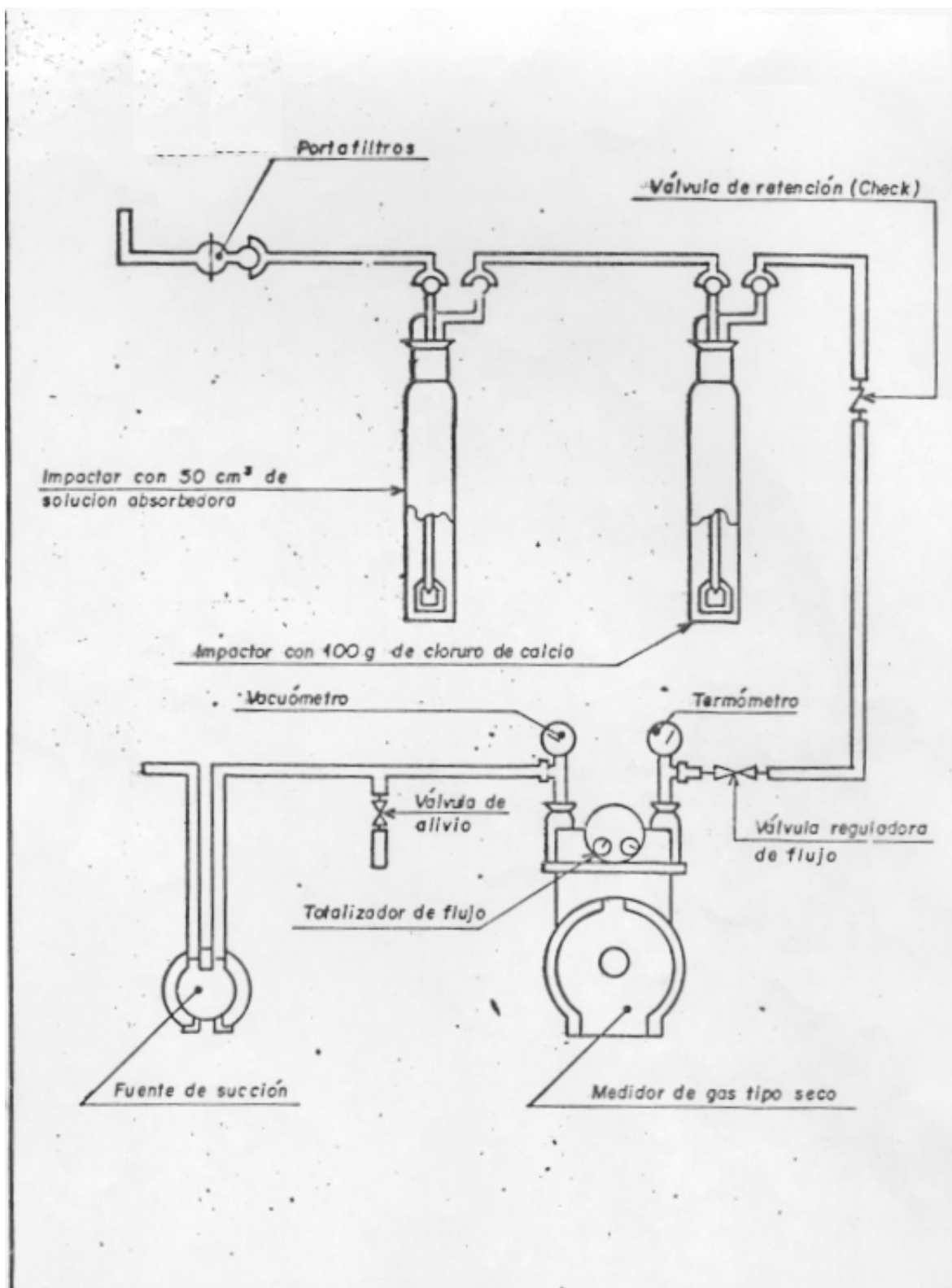
FIGURA 1 .- TREN DE MUESTREO PARA AMONIACO
