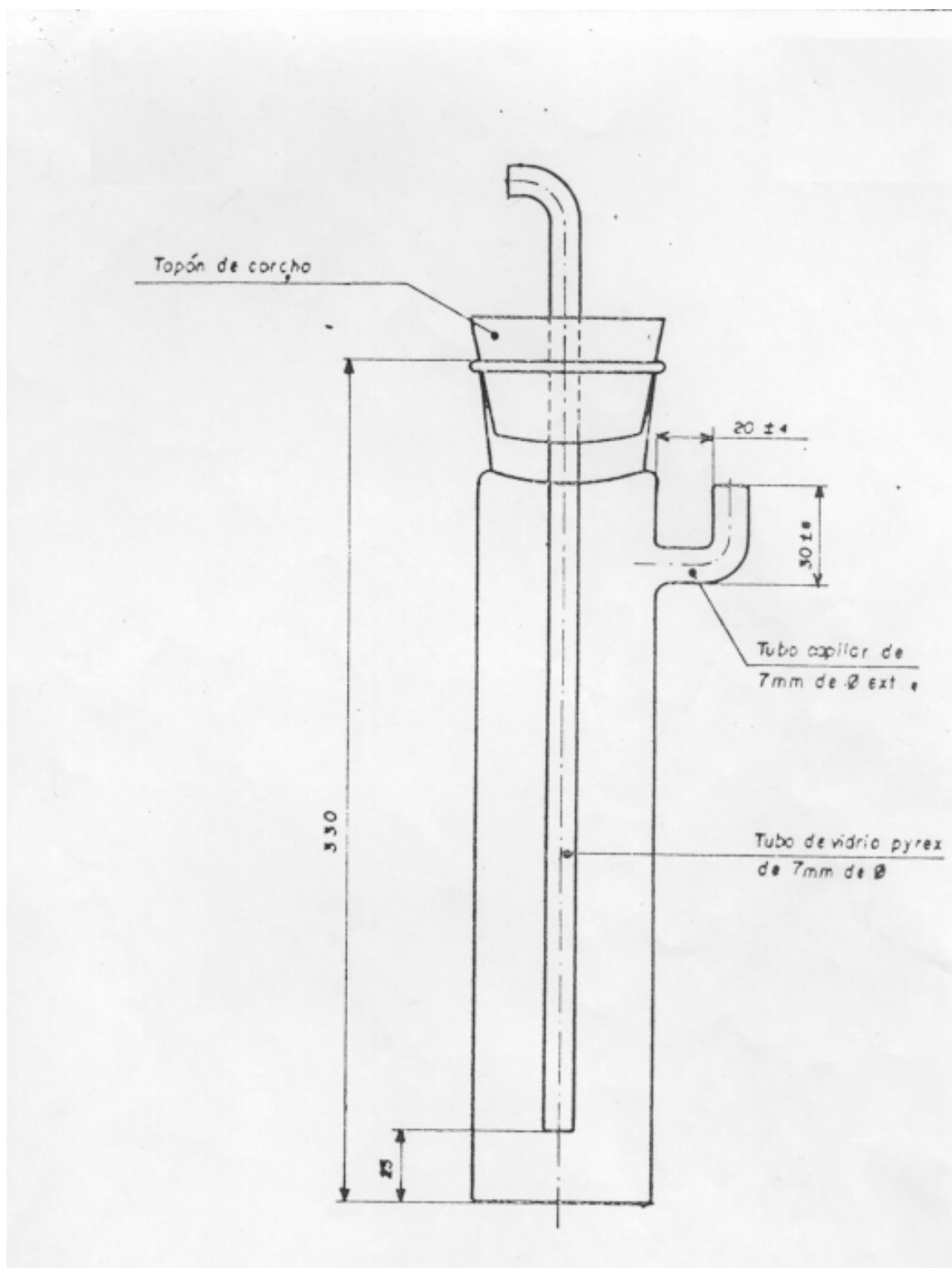
FIGURA 2: BURBUJEADOR NORMAL
